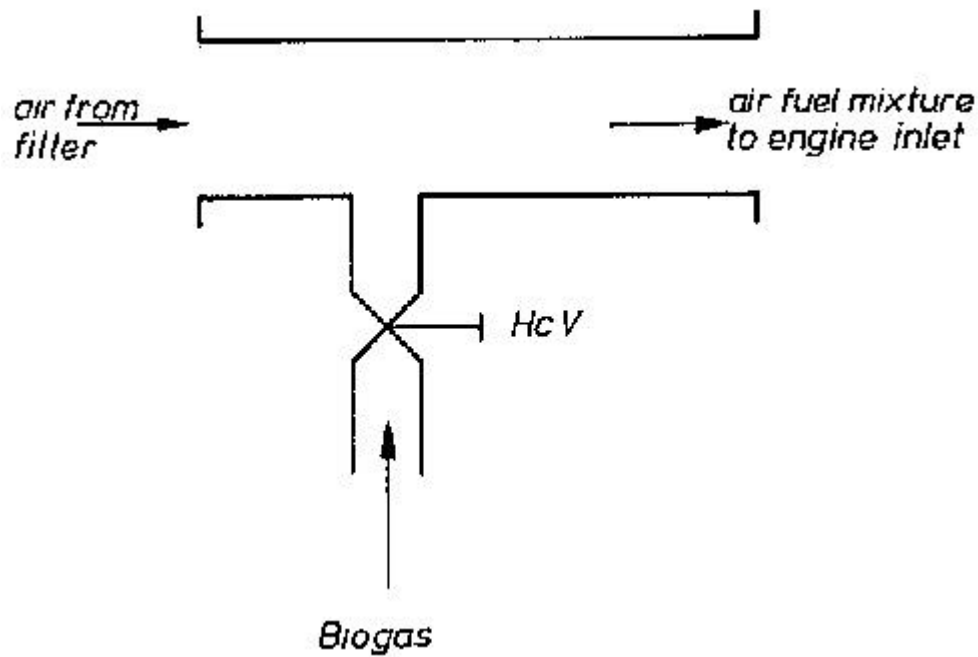
Fig. 5.1: T-joint mixer
