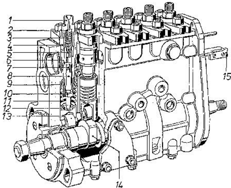
Fig. 3.11: Diesel injector pump (Bosch).
