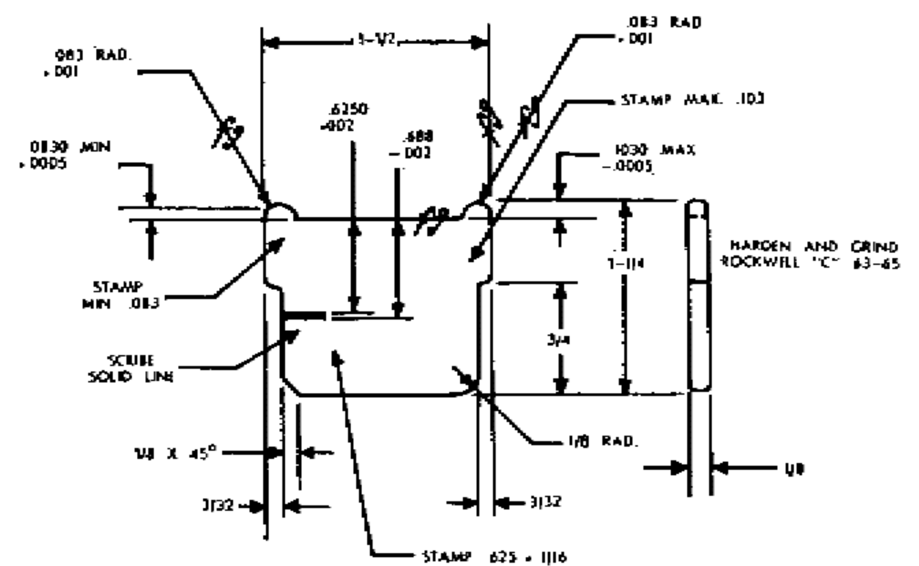
Fig. 110. Depth gage.
