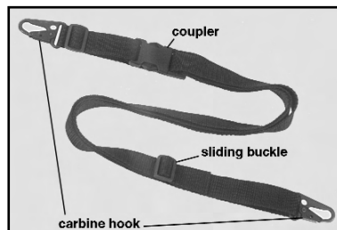
Fig. 14 Sling
